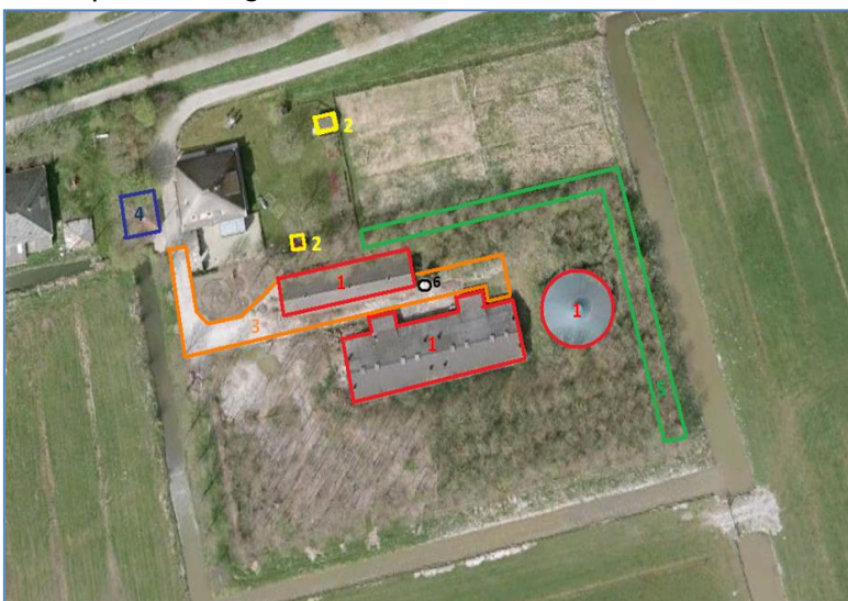
Afbeelding 3. huidige situatie met overzicht te saneren bouwwerken/ verhardingen (bron: Google Earth)
